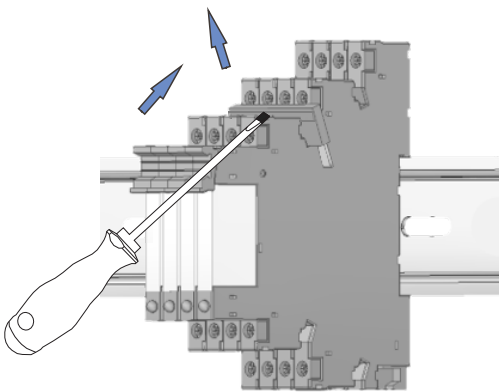
Extracción / Extraction
